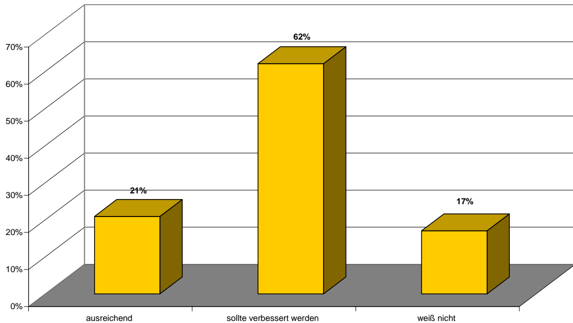
Abb. 4.18: Informationsbedarf in %.
