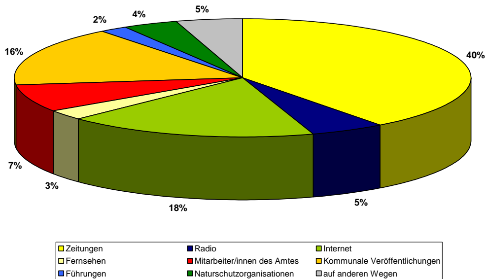
Abb. 4.17: Informationsmedien in %.
