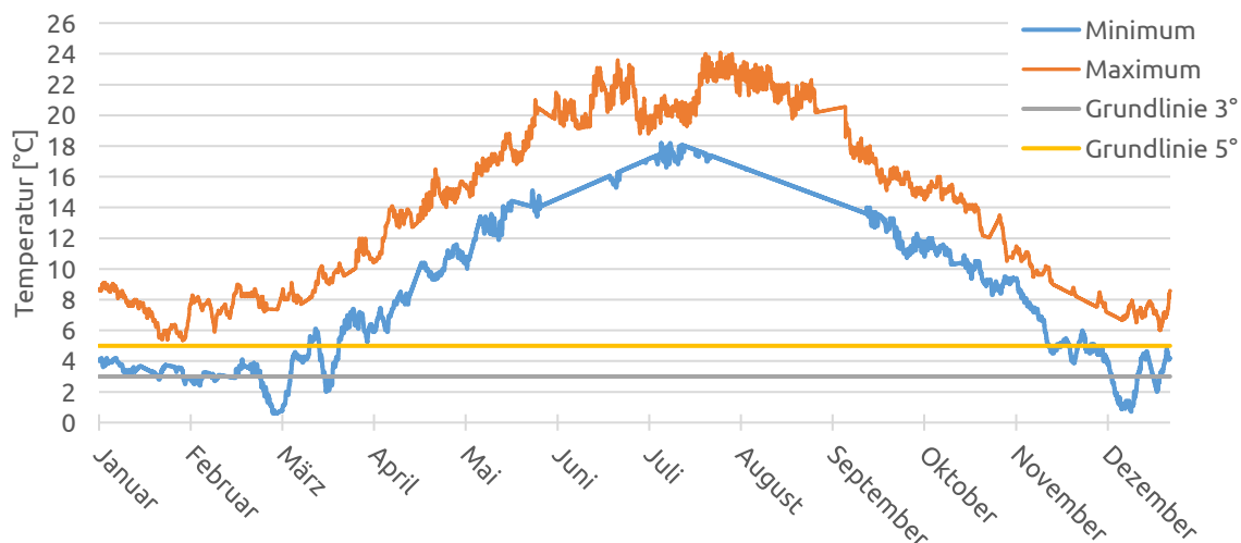
Abbildung 15: Interpolierter Temperaturverlauf der Oker in den Jahren 2018 bis 2024
