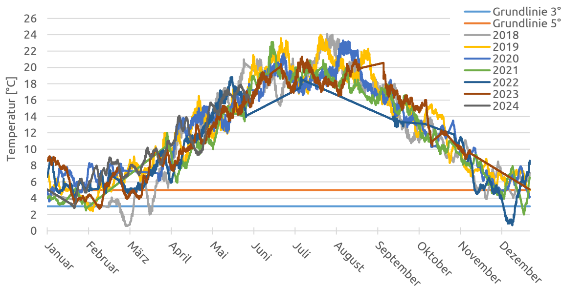
Abbildung 14: Interpolierter Temperaturverlauf der Oker in den Jahren 2018 bis 2024
