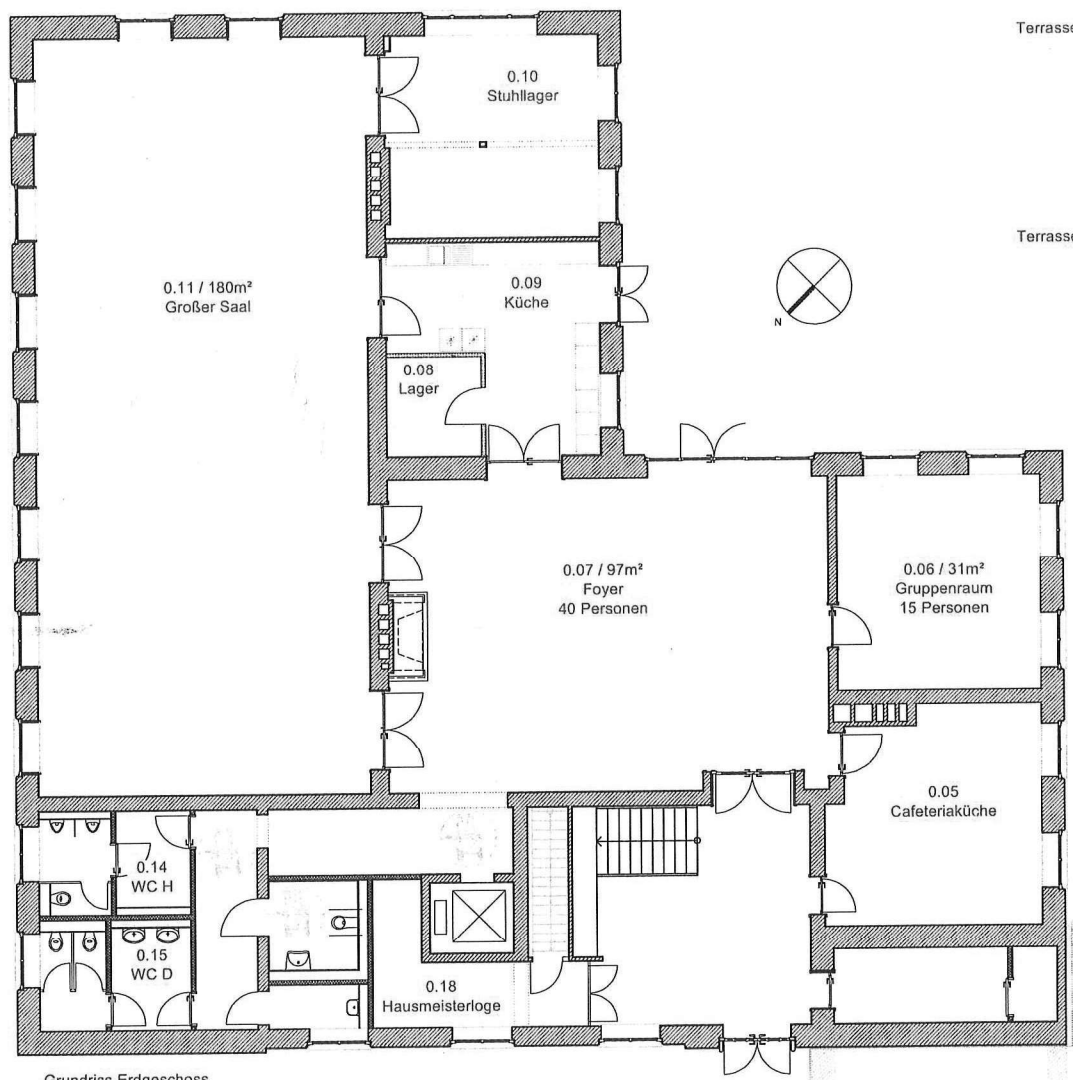
Grundriss Erdgeschoss
