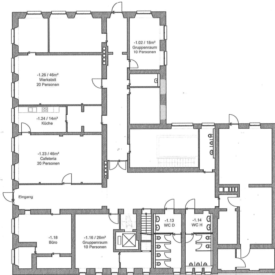
Grundriss Untergeschoss
